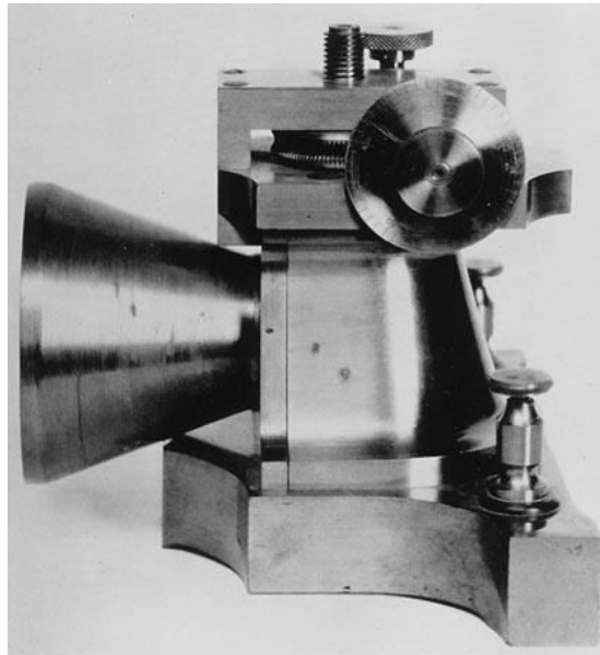
Edison tágulós hőmérője. A tölcser (balra) kb. 7 cm átmérőjű. ( www.americanscientist.org )
